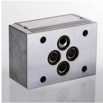
Modelis Starpplātņu vārsts Eksploatācijas spiediens maks. 350 bar Savienojums ISO/Cetop 03 size 6
